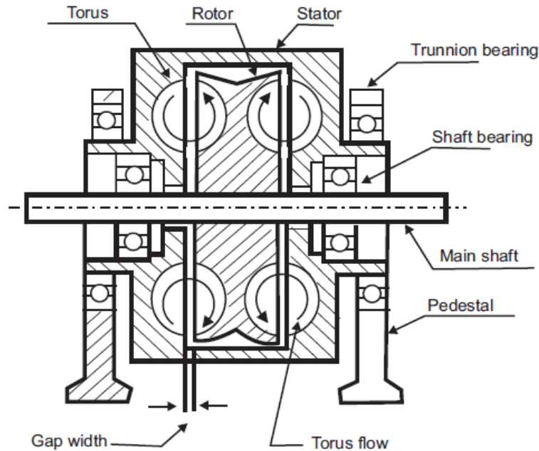
Fig. 31. Hydraulic dynamometer
